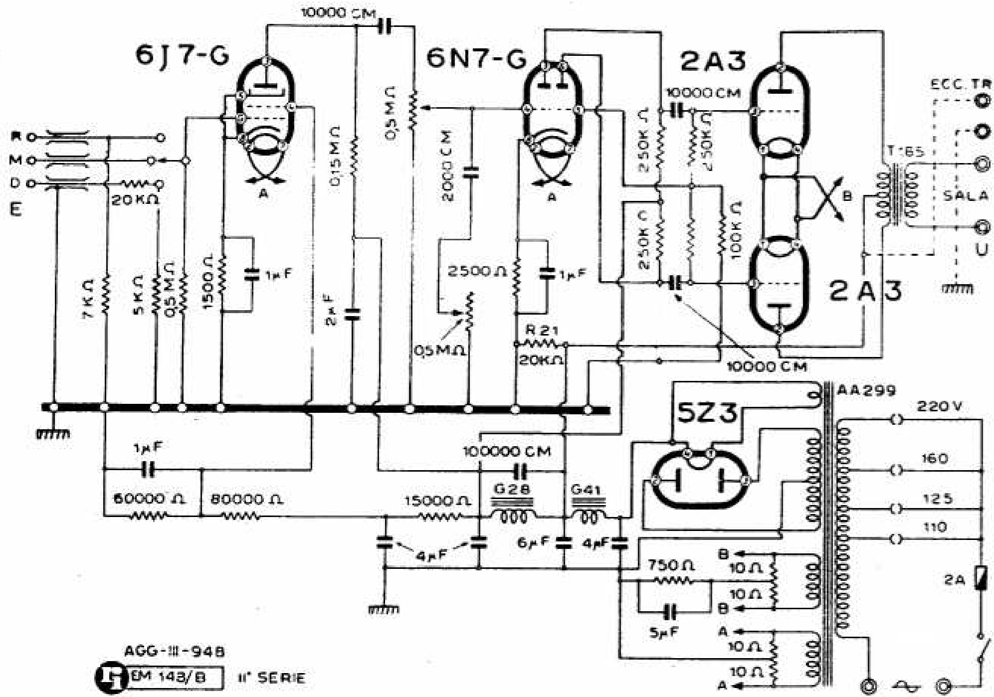
Allocchio Bacchini Amplificatore Albi 12 II serie
